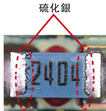
硫化贴片电阻
