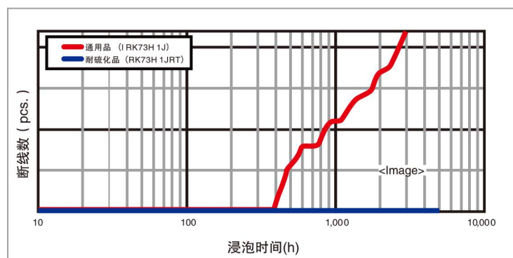
硫化试验结果 硫黄成分3.5%含有工业用油浸渍
