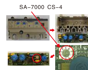
漏电保护器
