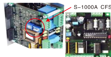
步进马达控制板
