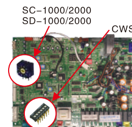
空调控制板
