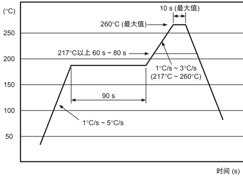
图6 耐热性评价用回流温度变化曲线
