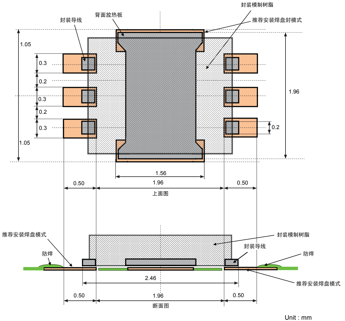
图4 HSNT-6A封装推荐安装焊盘与封装的位置关系
