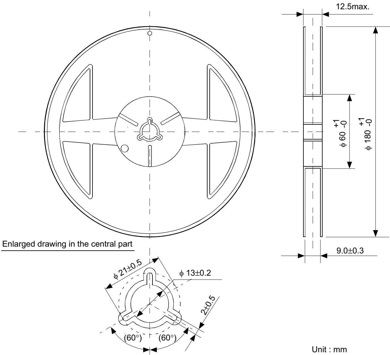
图11 HSNT-6A封装的带卷图面
