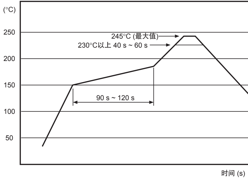
图5 安装性能评价用回流焊温度变化曲线
