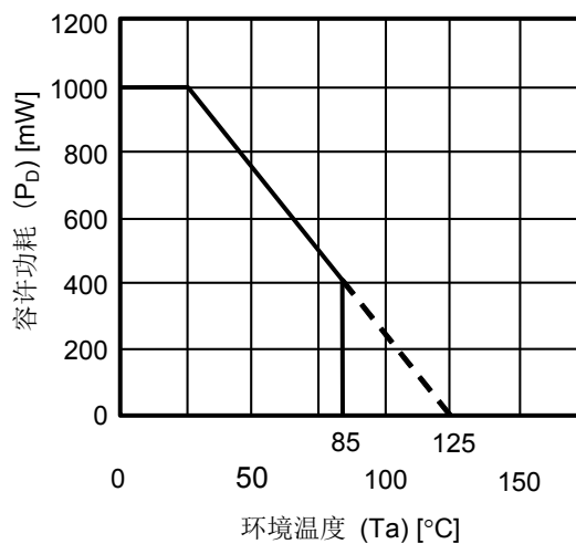
图7 HSNT-6A封装的容许功耗
