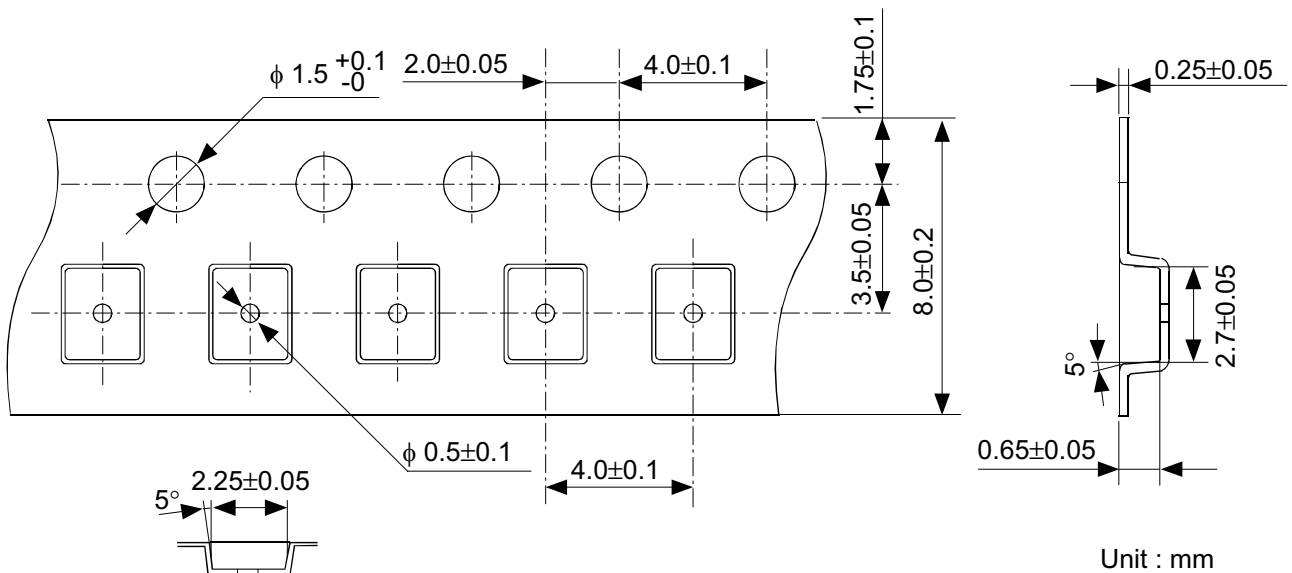
图10 HSNT-6A封装的卷带图面
