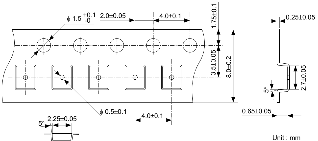
图27 SNT-8A的卷带图面
