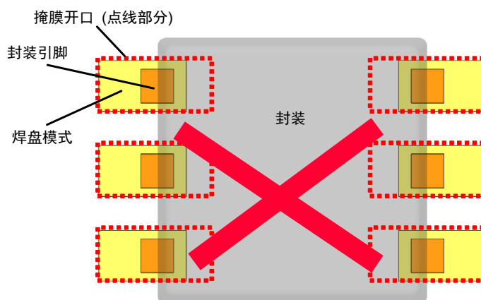
图13 掩膜开口向引脚内侧扩展示例 (不良品示例)
