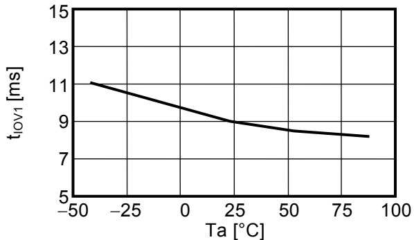
过电流1检测延迟时间—温度特性
