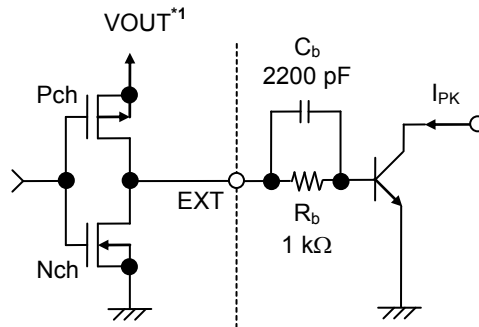
图 20 外接晶体管外围电路
