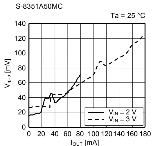
图16 输出电流( I_{OUT} ) — 纹波电压( V_{rp-p} )特性
