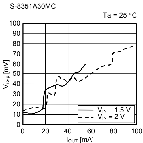
图15 输出电流( I_{OUT} ) — 纹波电压( V_{rp-p} )特性
