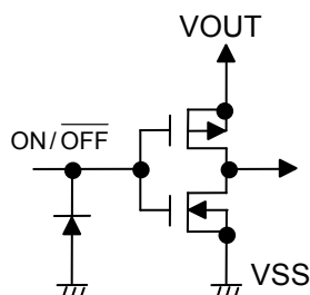
图 17 ON/OFF 端子的构造
