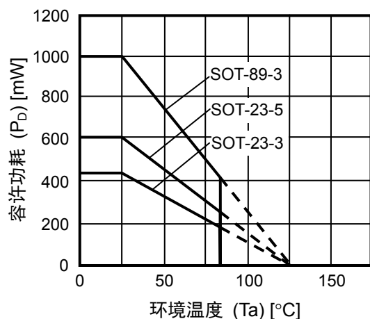
(1) 基板安装时
