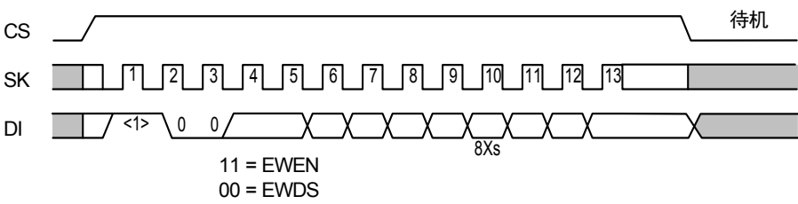
图11 允许或禁止写入定时
