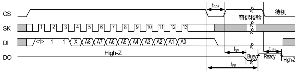
图8 数据删除定时
