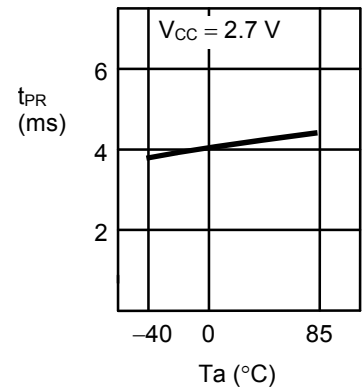
2.5 写入时间 t_{PR} —环境温度 T_a
