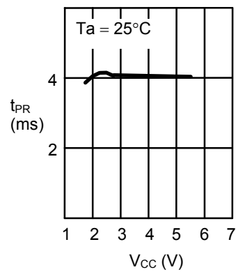
2.2 写入时间 t_{PR} —电源电压 V_{CC}
