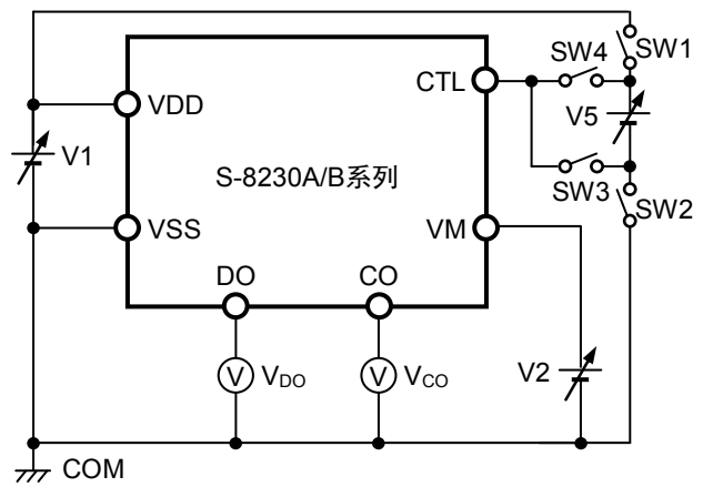
图5 测定电路2
