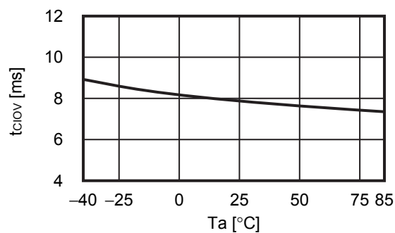
3.7 t_{CIOV} - T_a
