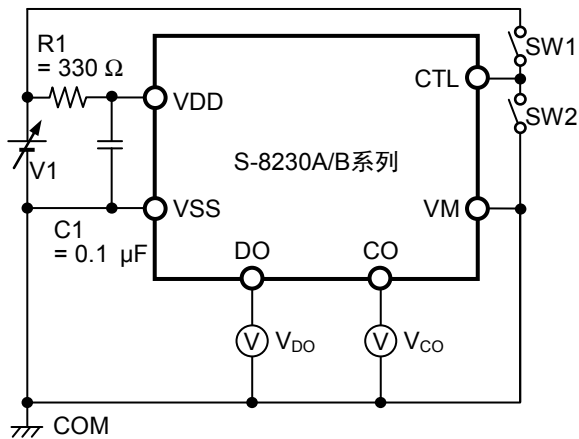
图4 测定电路1
