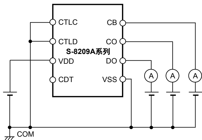
图13 测定电路7
