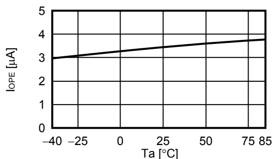
1.1 I_{OPE} - T_a
