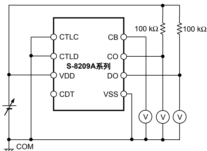
图7 测定电路1
