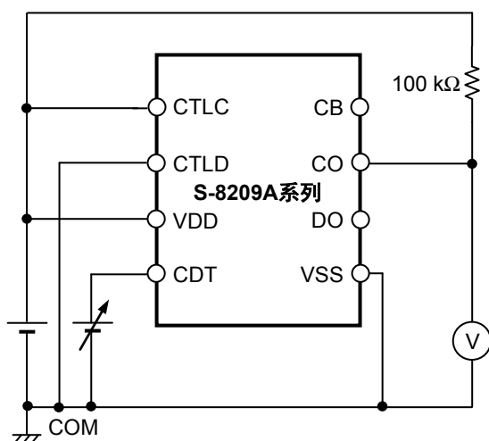
图9 测定电路3
