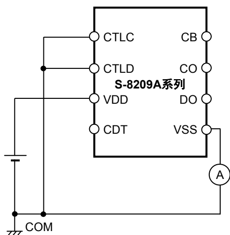
图11 测定电路5
