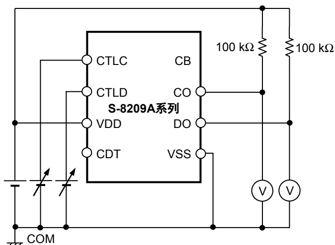
图10 测定电路4
