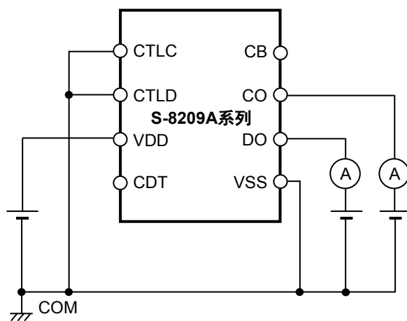
图14 测定电路8
