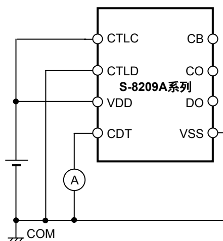
图8 测定电路2
