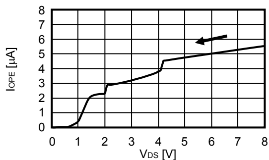
1.2 I_{OPE} - V_{DS}
