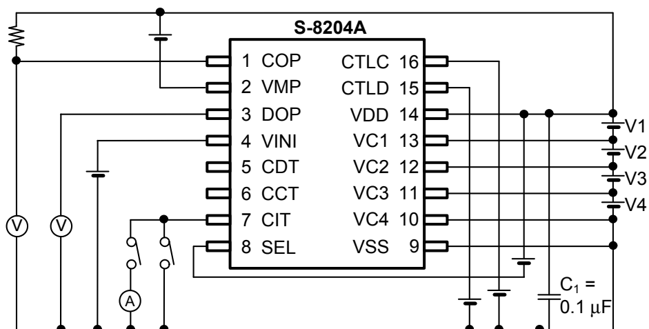
图5 测定电路2
